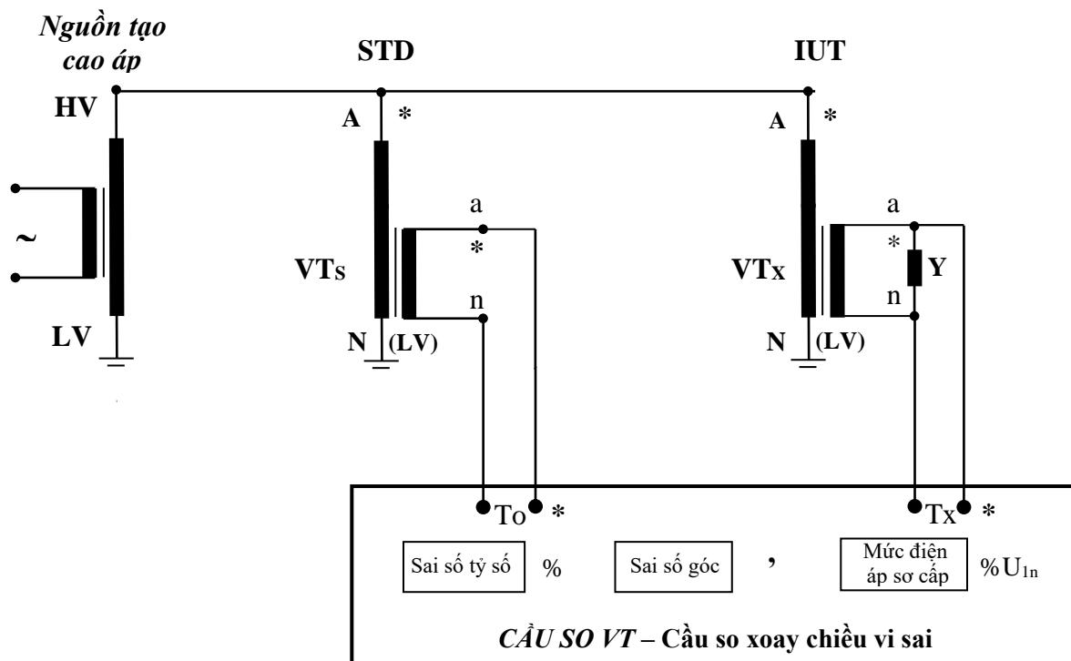
Hình 1. Sơ đồ mạch kiểm định biến áp đo lường
